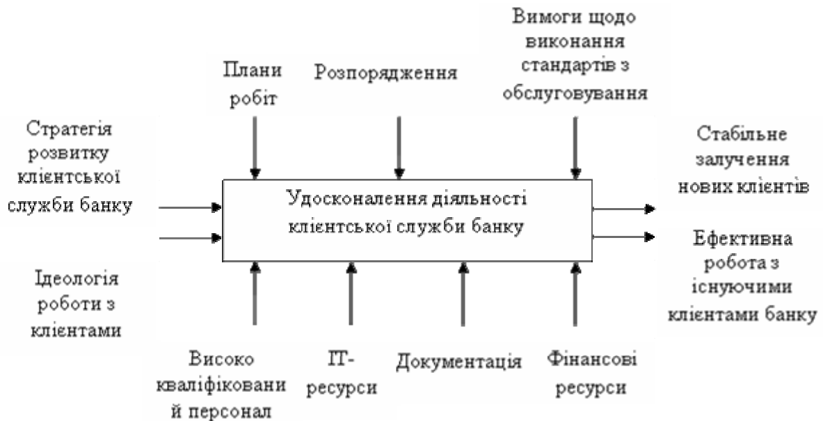
Рис. 3. Контекстна діаграма SADT-моделі вдосконалення діяльності клієнтської служби
